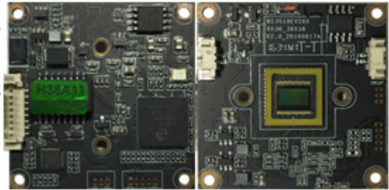
38 单板, 200 万, 低照, 低码流, 低功耗, IR-CUT 驱动, 3D 降噪, H. 264+
